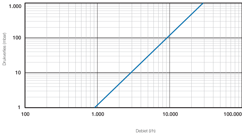
Drukverliescurve HK 40/50
