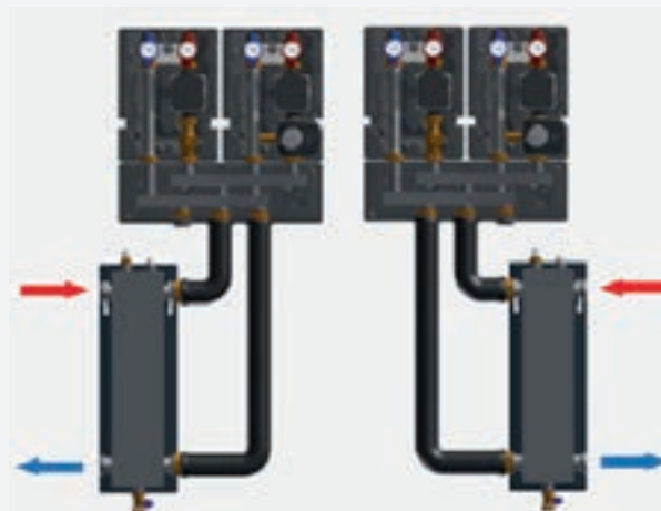
Flowbox installatie met HW evenwichtsfles en RB-HW buizenet:
