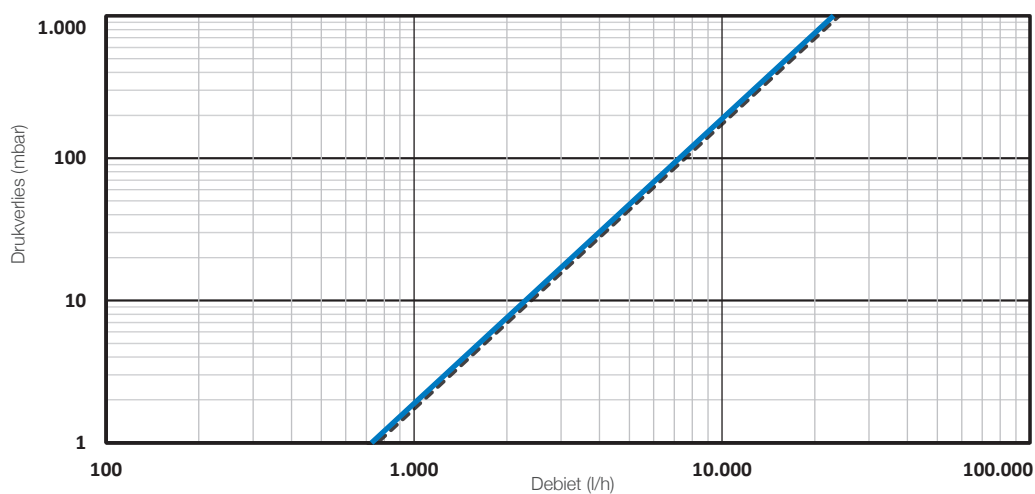
Drukverliescurve HK 40/50
