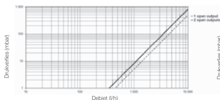
Drukverliescurve VB 20-2
