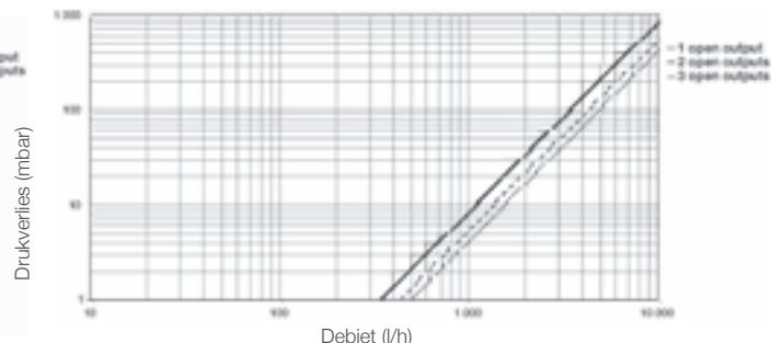
Drukverliescurve VB 20-3
